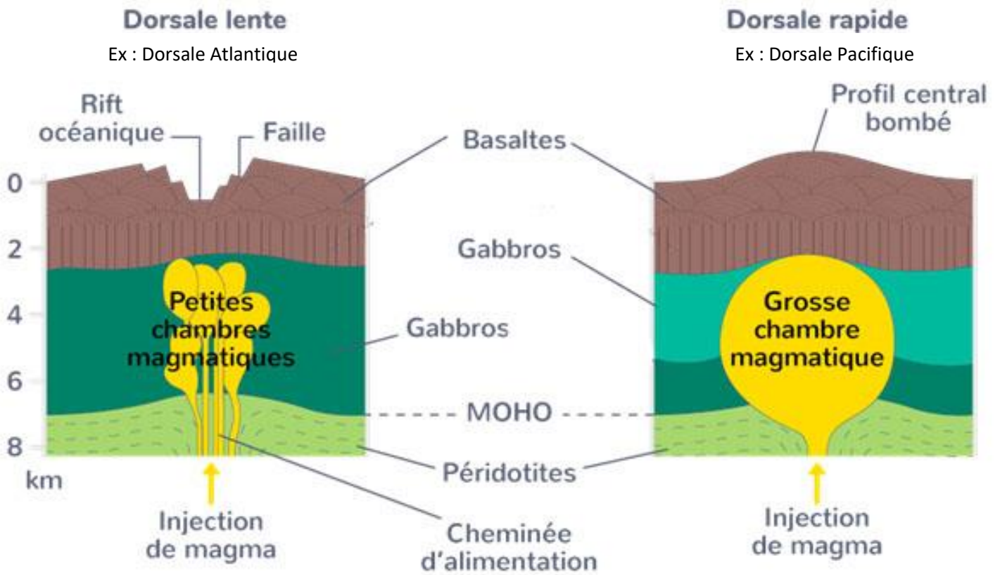
Schéma Bilan : Dorsale rapide et dorsale lente.
