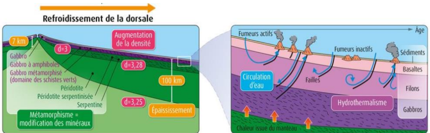
Schéma Bilan : L'Altération de la lithosphère océanique
